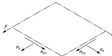
Bild 5. Scheibenschnittgrößen
