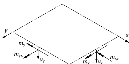
Bild 4. Plattenschnittgrößen
